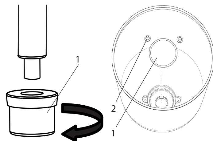
système d'aspiration
