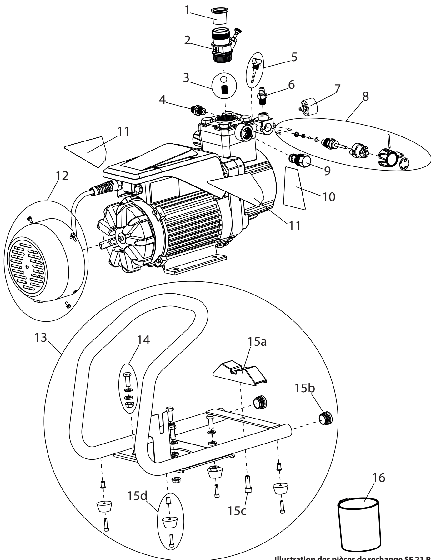
Illustration des pièces de rechange SF 21 Pro
